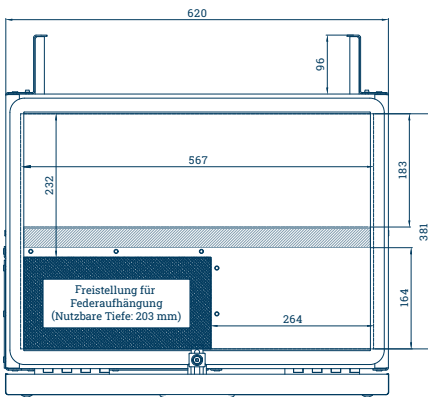
UnterflurBox UB-62: Beifahrerseite, mit Zwischenboden, Maße in mm
