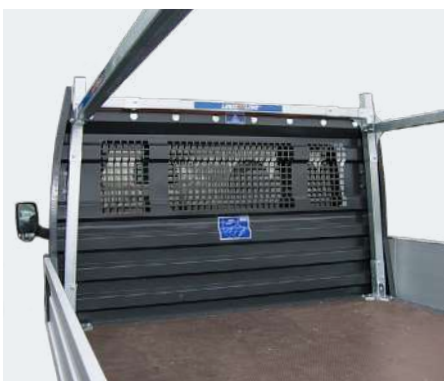
PowerRack auch bei Ford Transit möglich: Montage hinter / zwischen dem werkseitigen Fahrerhausschutz
