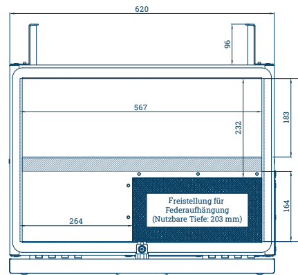
UnterflurBox UB-62: Fahrerseite, mit Zwischenboden, Maße in mm
