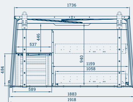
RB-125 / RB-150: Heckansicht mit opt. Auszugsladen und Ladencontainer
