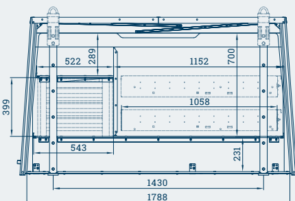
RB-125 / RB-150: Frontansicht mit opt. Auszugsladen und Ladencontainer
