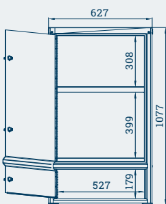
RoadBox RB-65: Fahrerseite, Beifahrerseite bis auf Beladetiefen und Türöffnungsrichtung identisch
