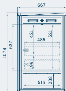
RoadBox RB-70: Ansicht Beifahrerseite mit opt. Auszugsladen
