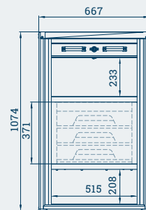
RoadBox RB-70: Ansicht Fahrerseite mit opt. Ladencontainer
