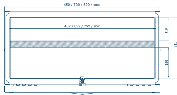
UnterflurBox UB-45 / UB-70 / UB-80 / UB-100: mit Zwischenboden, Maße in mm
