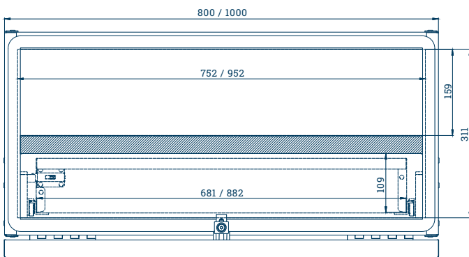
UnterflurBox UB-80 / UB-100 mit Auszugslade und Zwischenboden, Maße in mm
