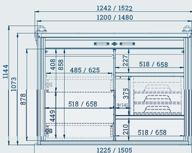
RB-125 / RB-150 Beifahrerseite mit opt. Auszugsladen und Ladencontainer
