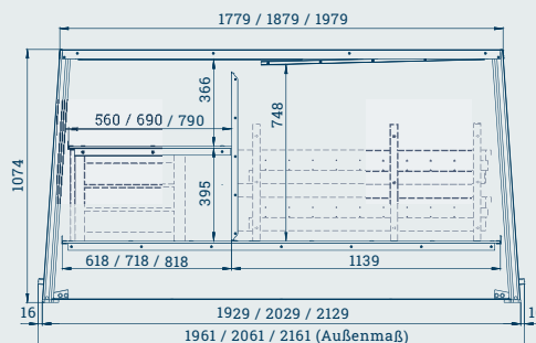
RoadBox RB-70: Heckansicht, RoadBox mit optionalem Zubehör
