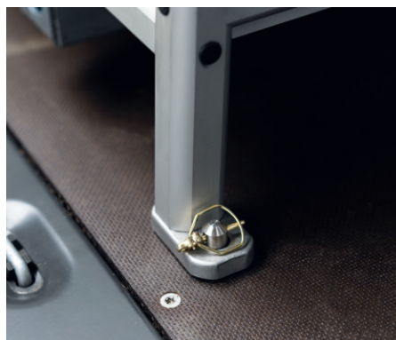
Schnellmontagesystem* zur einfachen, werkzeuglosen Montage und Demontage der Box auf der Pritsche
