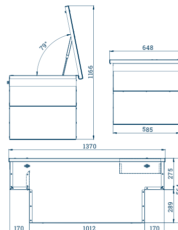
PickUp Box auf Ladefläche, in beladenem Zustand mit Fachteiler*
