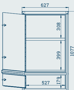
RoadBox RB-65: Ansicht Fahrerseite
