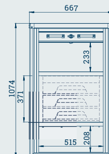
RoadBox RB-70: Ansicht Fahrerseite mit opt. Laden- container
